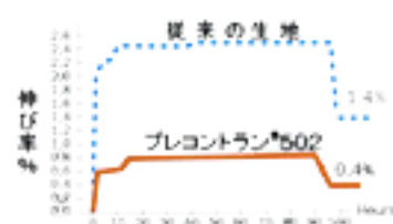
ヨコ方向における伸び率 (グラフ1)
